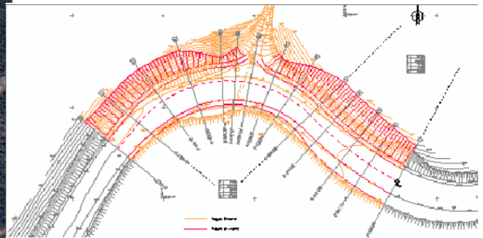
Fig. 1 – Planta do troço a intervir
