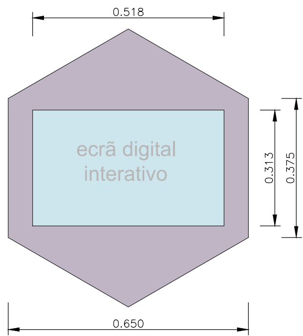
PLANTA DO TAMPO
