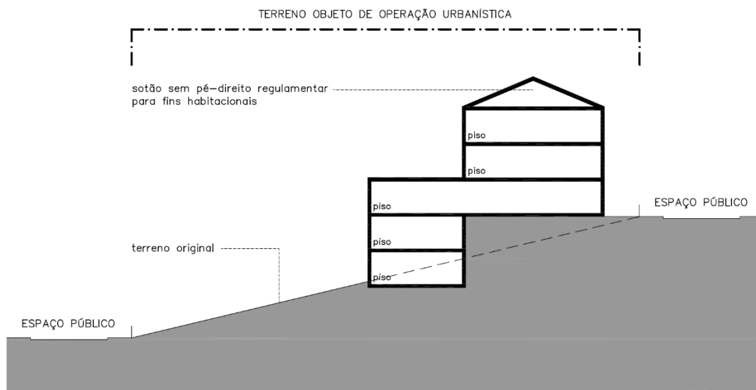
EXEMPLO 2 – 5 PISOS
