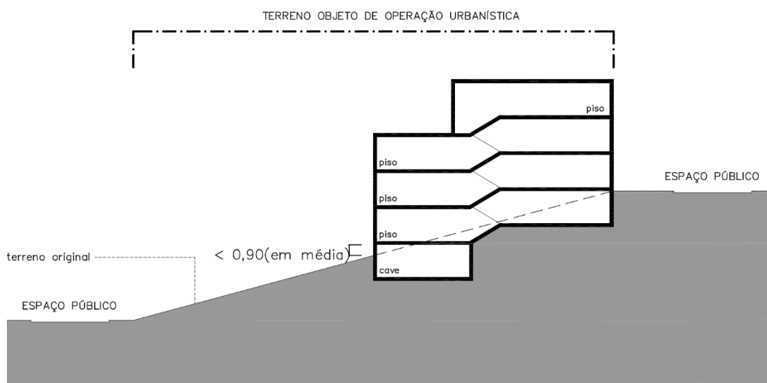
EXEMPLO 3 – 4 PISOS
