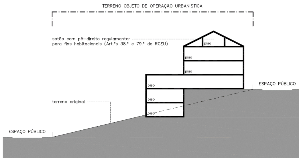
EXEMPLO 1 – 6 PISOS
