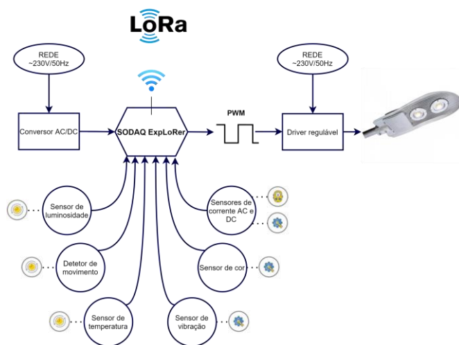
Fluxograma de controlo de cada luminária
