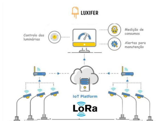
Interligação entre a aplicação e a luminária
