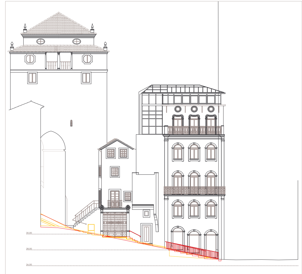
PERFIL B
